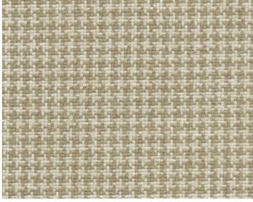
Llama
